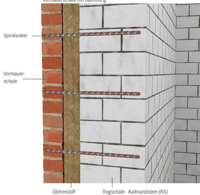
Vormauerschale mit Dämmung
