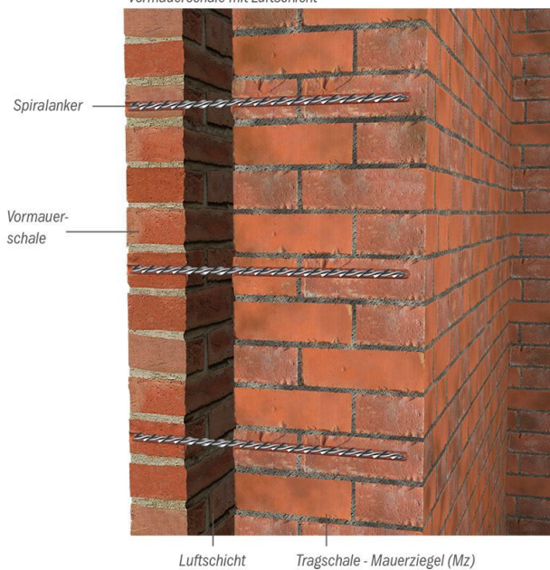
Vormauerschale mit Luftschicht
